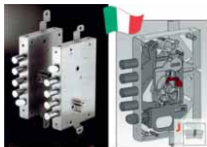
Κλειδαριά ISEO με καταπέλτη
